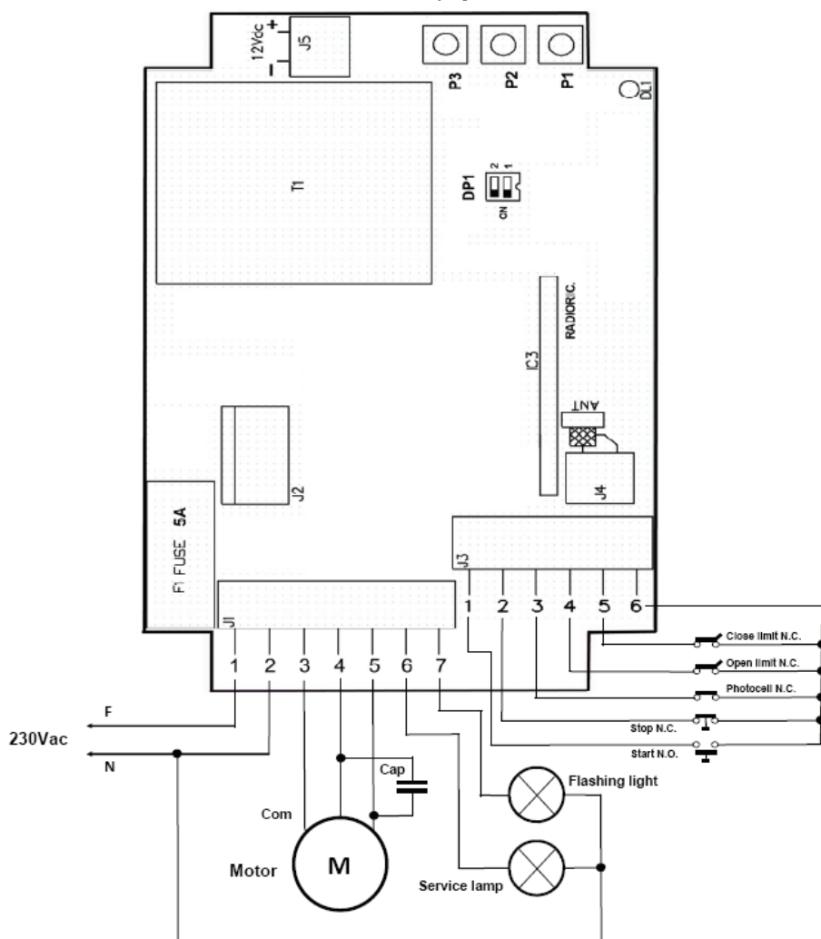
Nákres zapojení:
