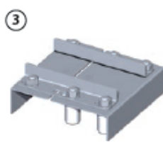
VA3501.A30/B40 komplet horního vedení vnitřního křídla
